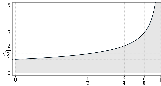
FIGURE 9.2 – Graphe de t \mapsto \frac{1}{\sqrt{1-t}} sur [0, 1[ . L'aire de la partie colorée est \int_0^1 \frac{dt}{\sqrt{1-t}} = 2 .
