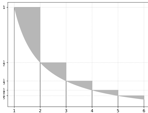
FIGURE 5.3 – Interprétation géométrique de la constante \gamma .
