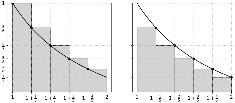
FIGURE 8.2 – A gauche, l'aire des rectangles est égale à S_5^+ . C'est aussi l'intégrale d'une certaine fonction en escaliers supérieure à f . A droite, l'aire des rectangles est égale à S_5^- .
