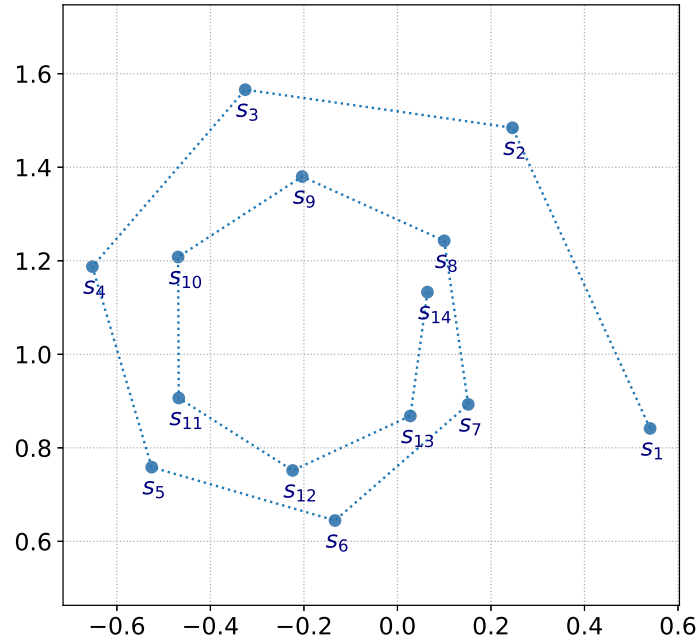
FIGURE 6.3 – Tracé dans le plan complexe de la somme partielle s_n = \sum_{k=1}^n \frac{e^{ik}}{\sqrt{n}} pour quelques valeurs de n .
