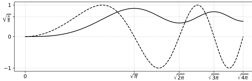
FIGURE 11.3 – Graphe de f : x \mapsto \sin(x^2) en pointillés et de F : x \mapsto \int_0^x \sin(t^2)dt en trait plein.
